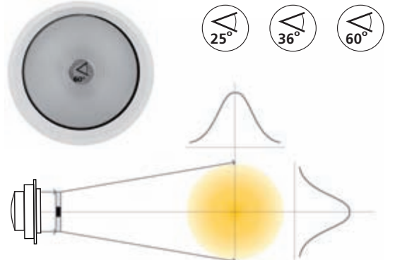
Dairesel ışık açılı filtre / Beam spreader snap
